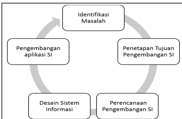
Gambar 1. Tahap Penelitian
