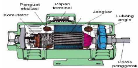
Gambar 8 Konstruksi Generator
