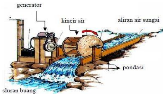
Gambar 1. Mikrohidro
