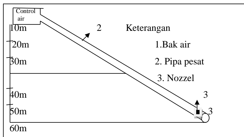
Gambar.3 Pipa pesat dan tinggi
